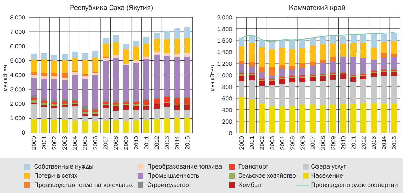
Рис. 2. Динамика и структура потребления электрической энергии в отдельных северных регионах
